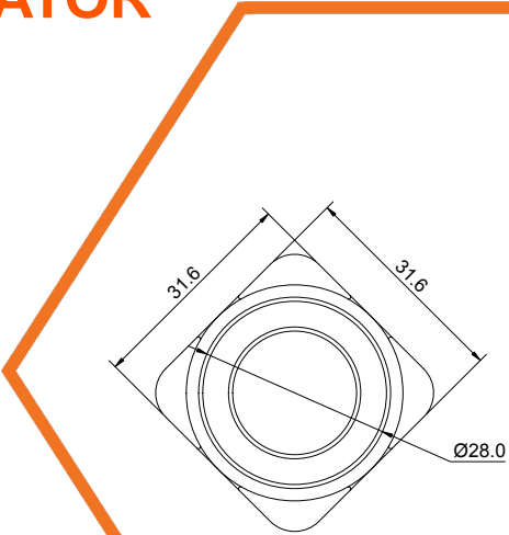
Dimensions Unit : mm Tolerance : ±0.3mm
