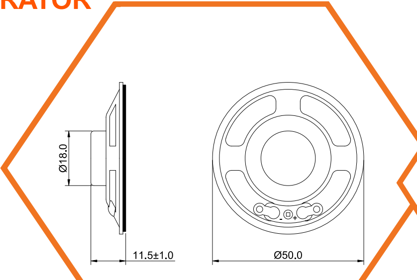
Dimensions Unit : mm Tolerance : \pm 0.3 mm
